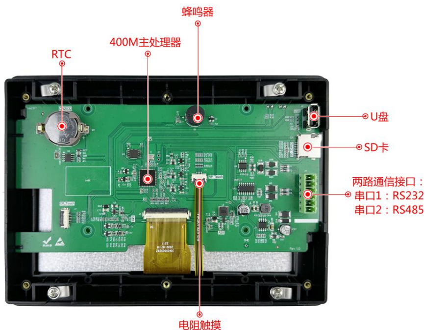
图 1-2 硬件配置图
