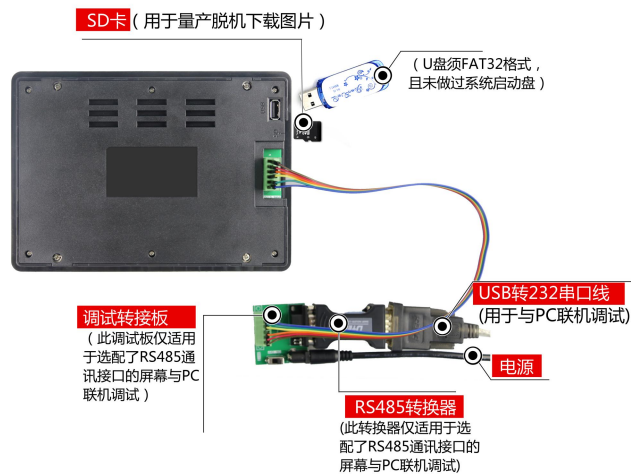
图 1-3 RS485 调试图
